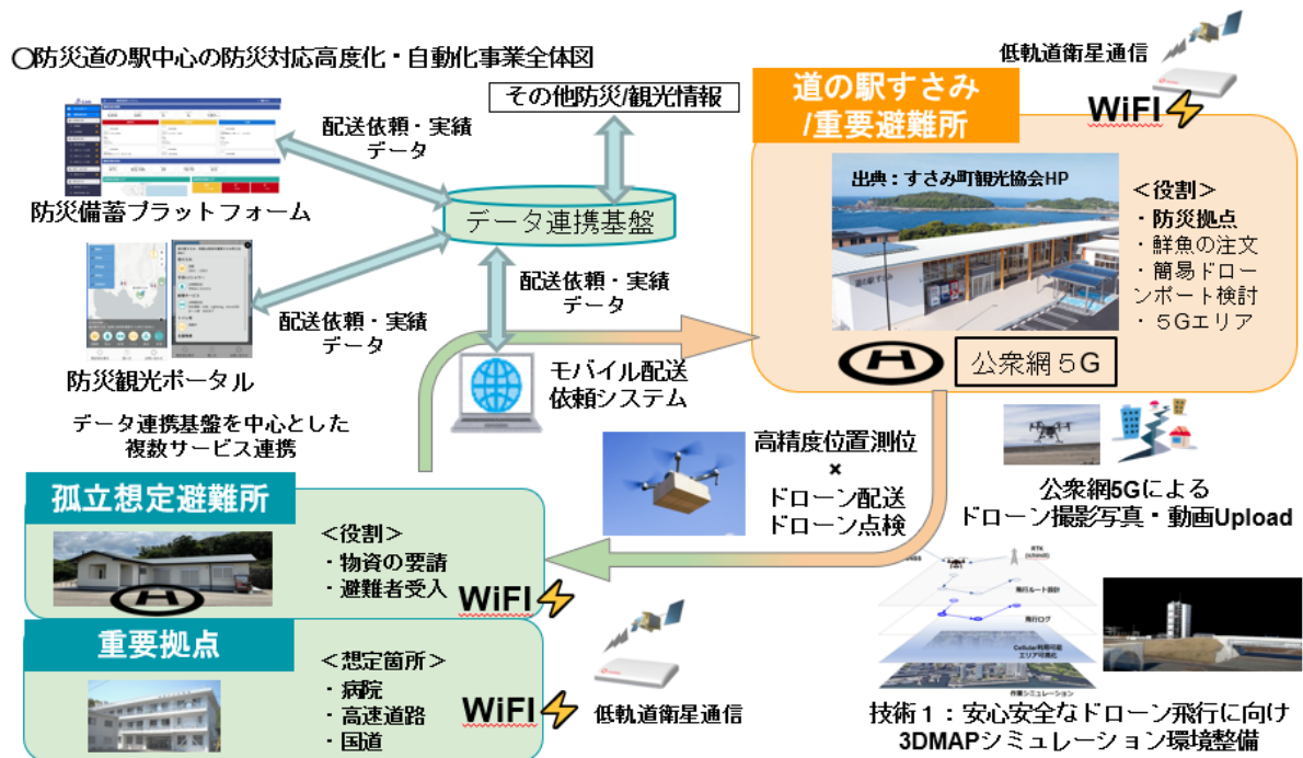
図表9 実証実験内容図解
